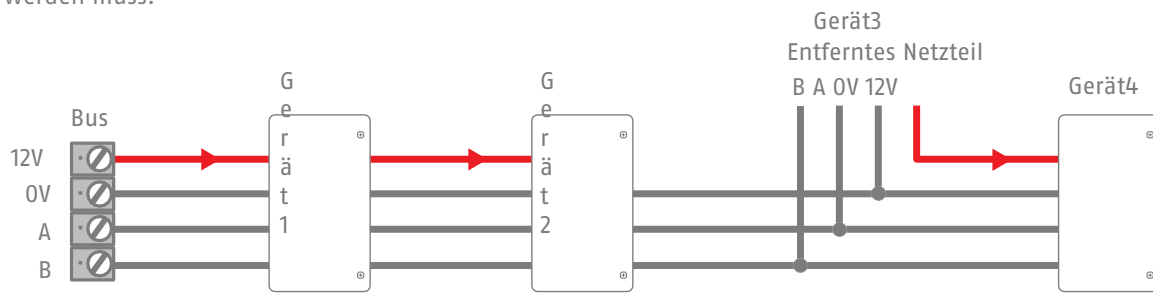
Abbildung 5: Anschließen einer externen Spannungsversorgung
