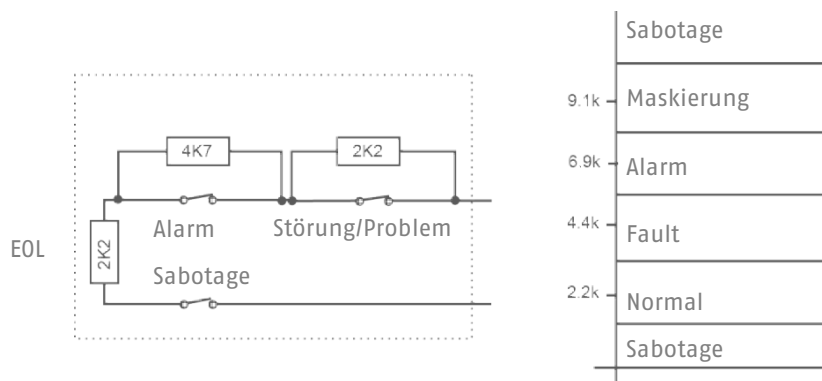
Abbildung 3: FSL-Anschlüsse mit Masking
