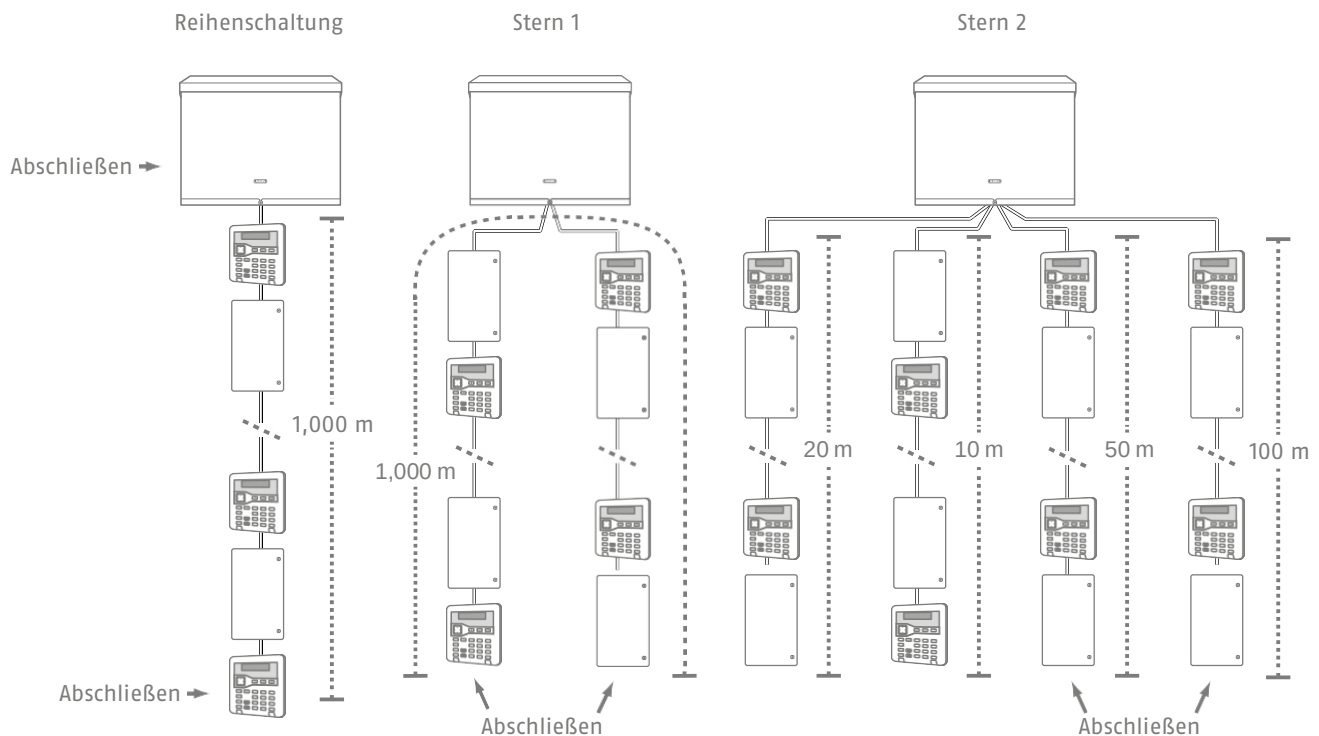
Abbildung 4: Busabschluss
