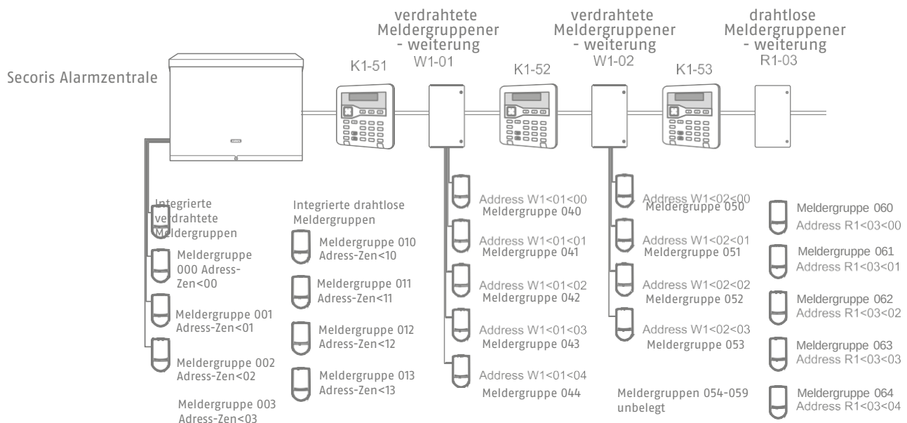
Abbildung 3: Beispiel für Melderadressierung und Meldergruppennummerierung
