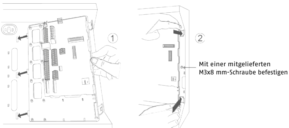
Abbildung 12: Secoris Alarmzentrale: Einbau der Platine
