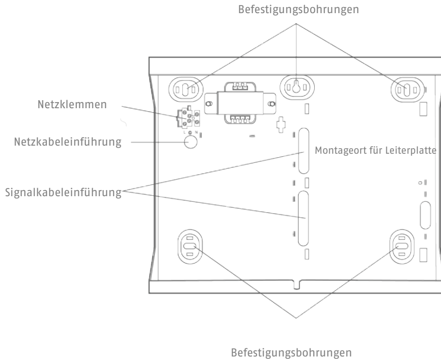
Abbildung 11: Secoris Alarmzentrale: Montagebohrungen und Kabeleinführungen
