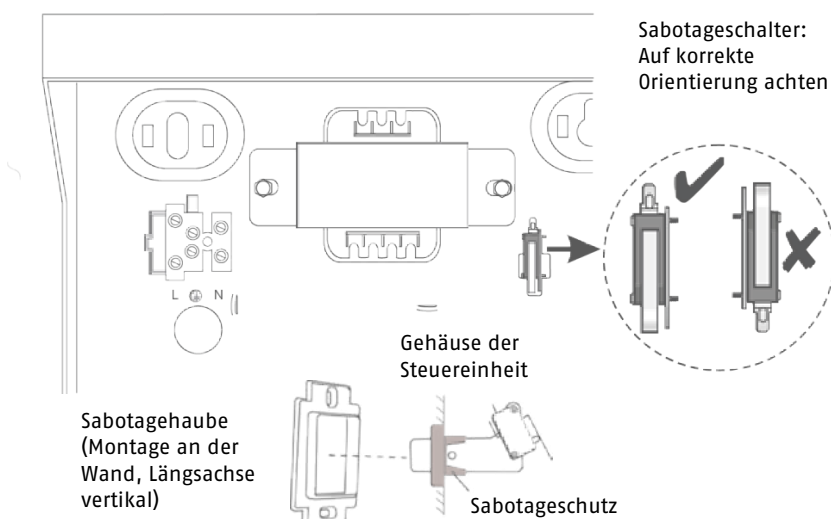
Abbildung 10: Secoris Alarmzentrale: Montage des Sabotageschalters und der Abdeckhaube
