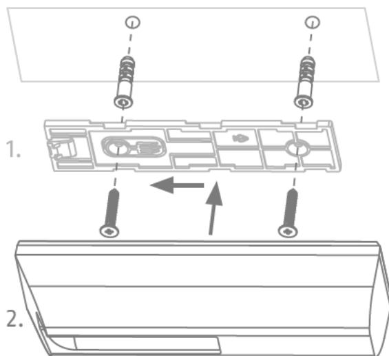
Montage directement au plafond
