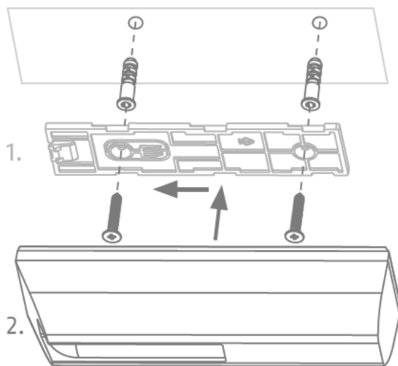
Montage direct aan het plafond
