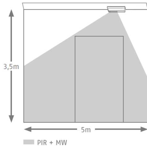
Montage direct aan het plafond
