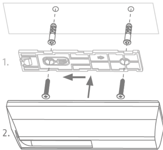
Montage direkt an der Decke
