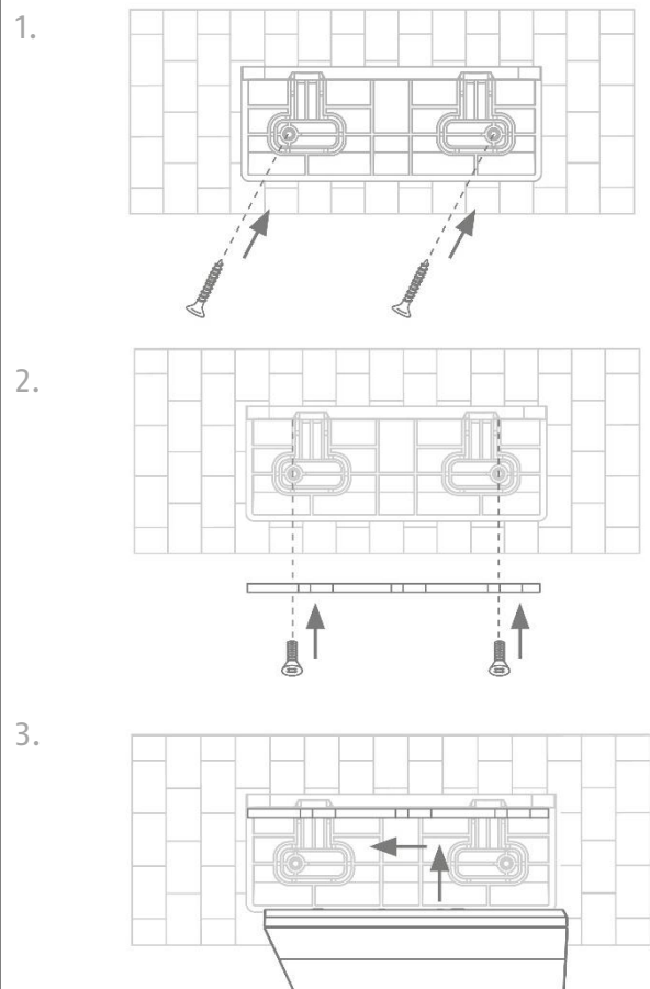
Montage avec support de montage en L à 90° sur le mur (détecteur vers le bas)
