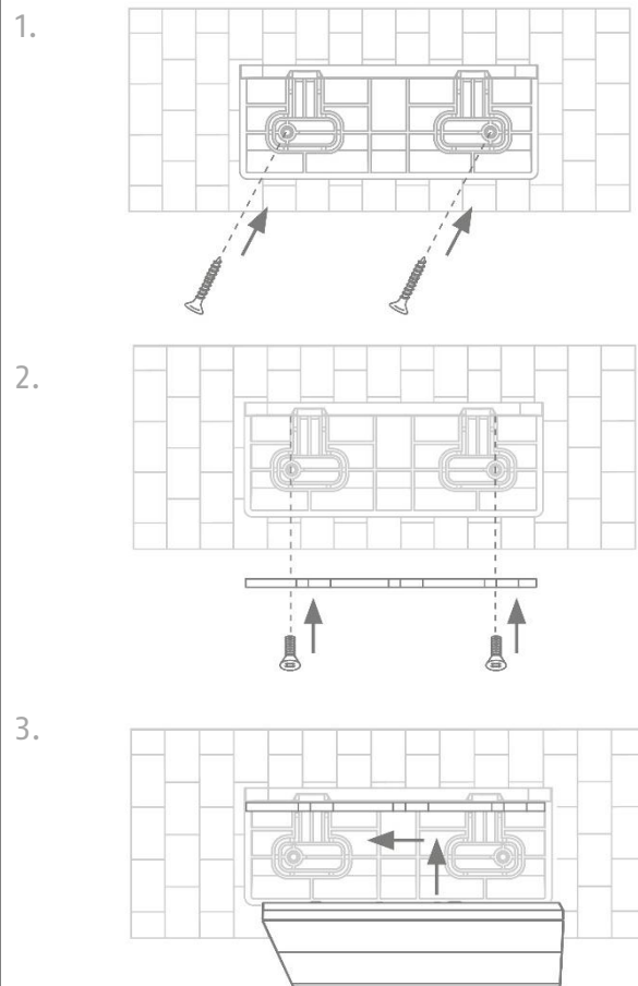
Montage mit 90° L-Montagehalter an der Wand (Melder nach unten schauend)
