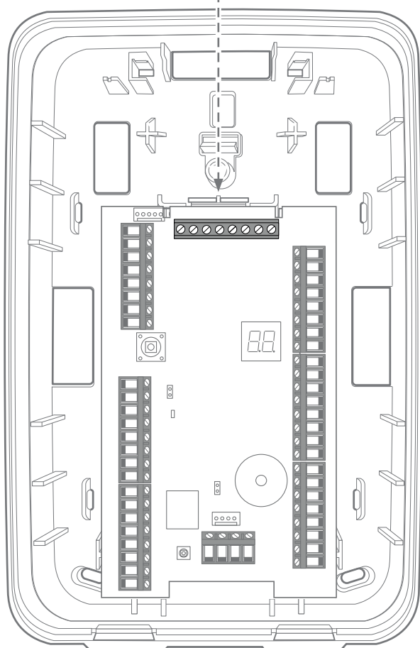
Abbildung 1: Secoris BUS-Drahterweiterung (10)
